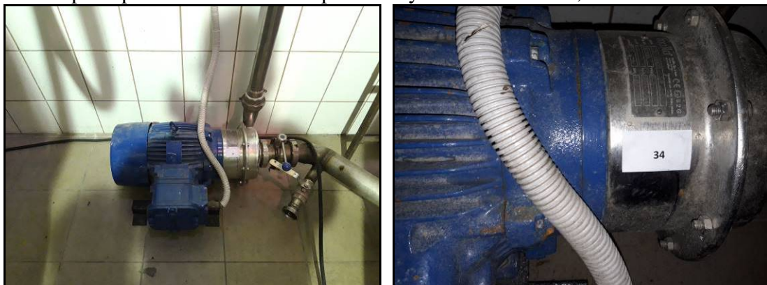
28. Pompa Tapflo CTDF-60X2D – przeciwybuchowa Silnik 7,5 kW
